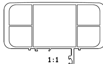
Obrázek vrchního madla - Rozměry 120x58x6 mm
