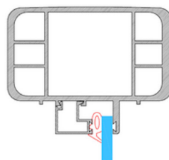
Řez madla zábradlí
