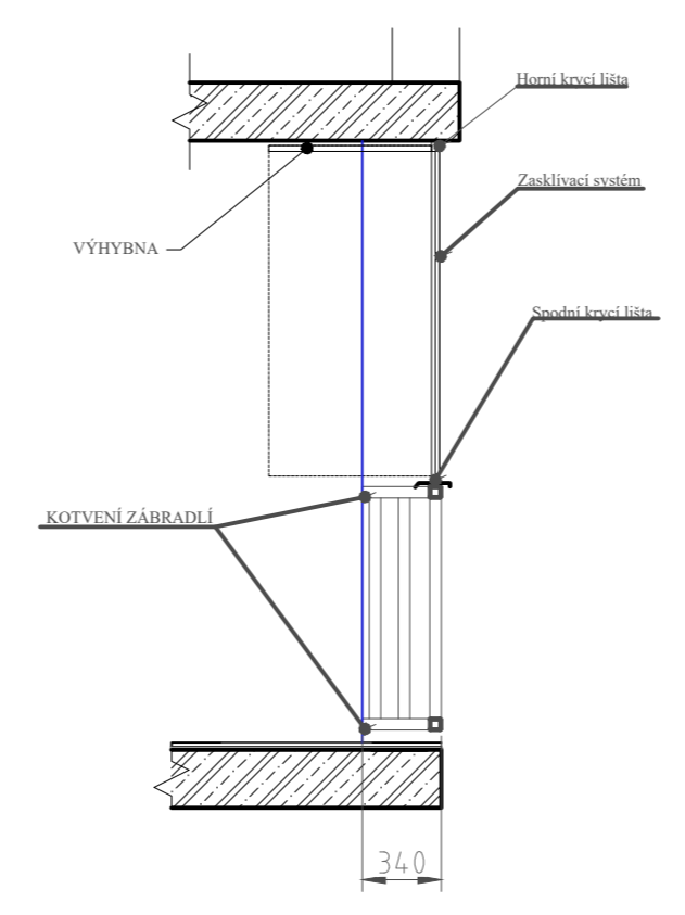
Řez
