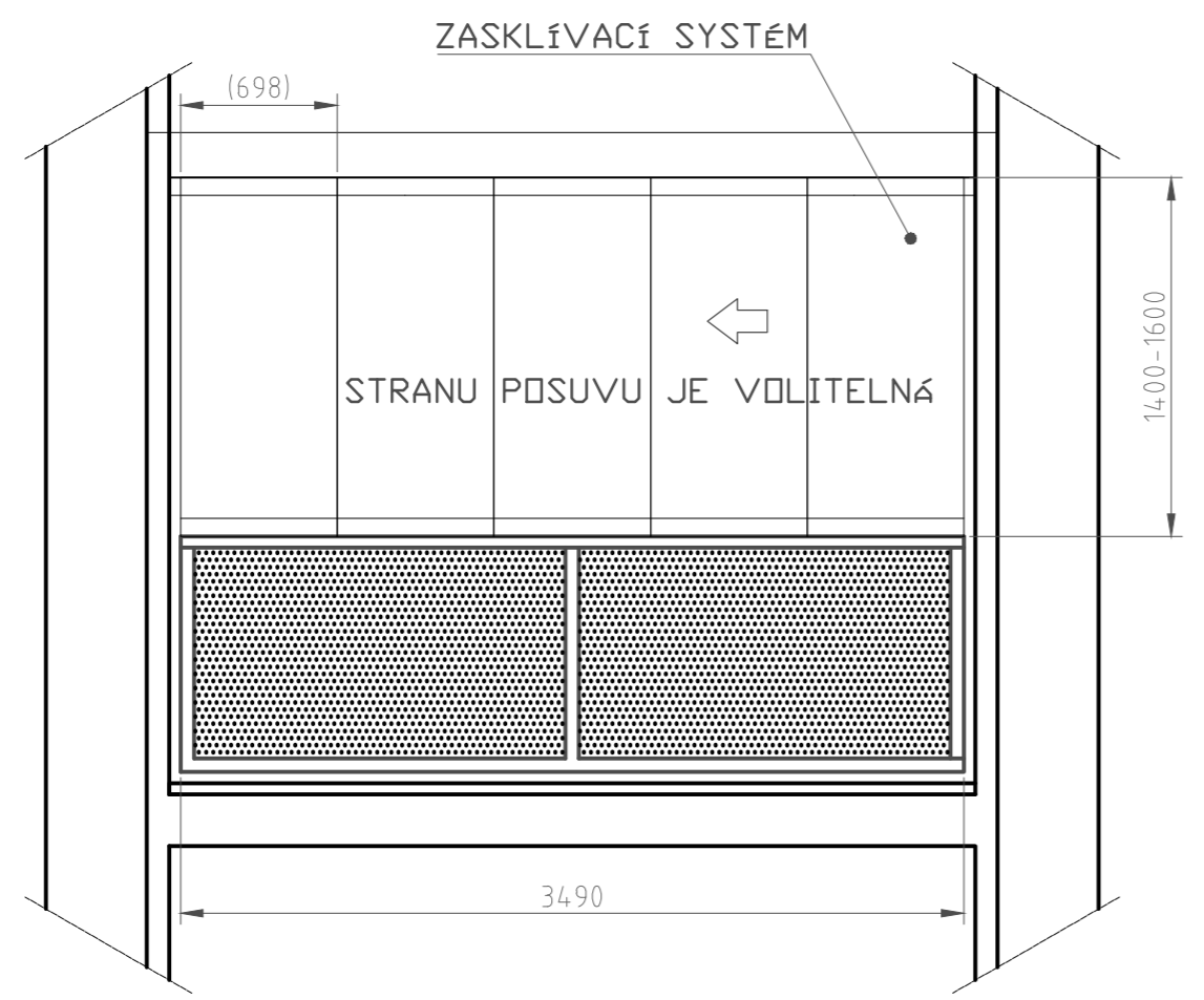
Pohled
