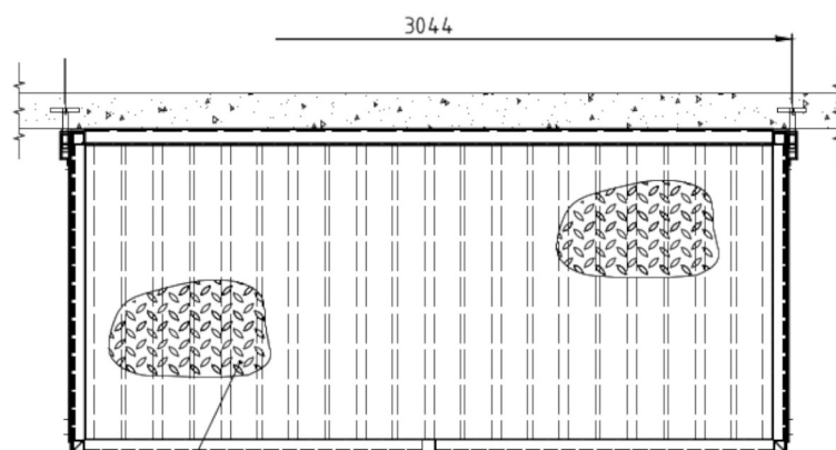
AL-SLZIČKOVÝ PLECH TL.4
