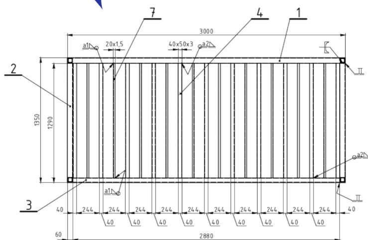
SVĚŘENEC PODESTY (ocelová konstrukce)
